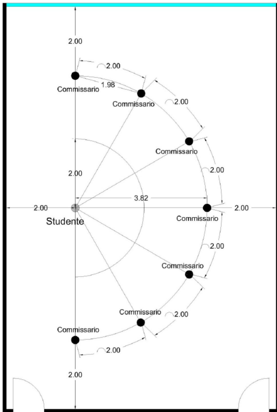
Parete finestrata - esemplificazione
